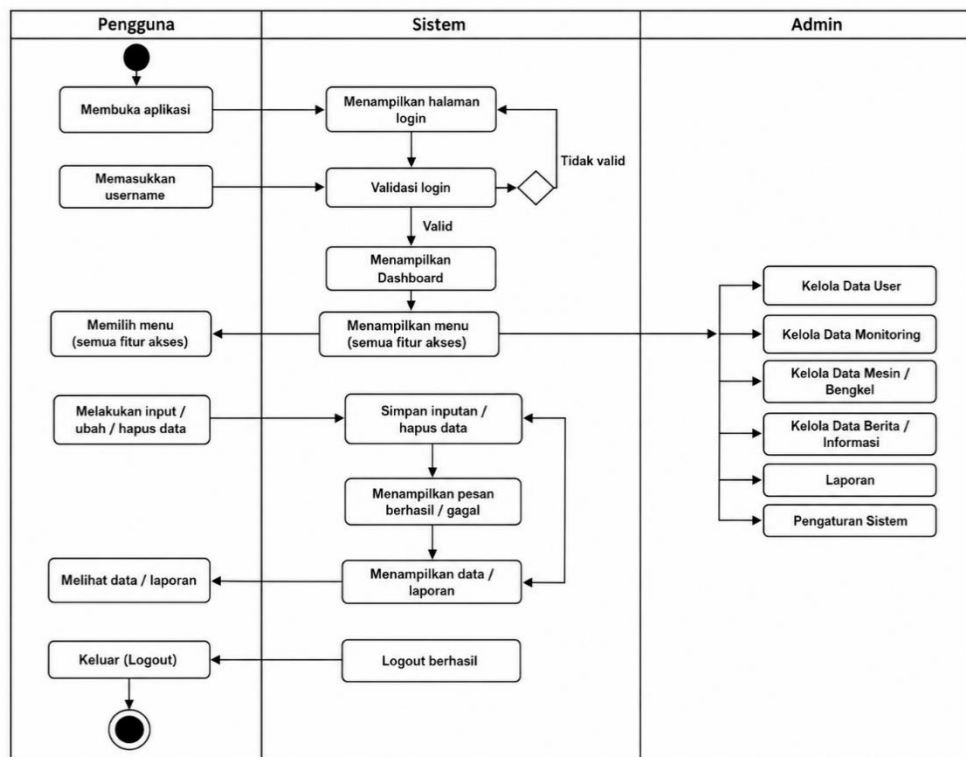
Gambar 4. Activity Diagram Sistem Manajemen Data Kakao
