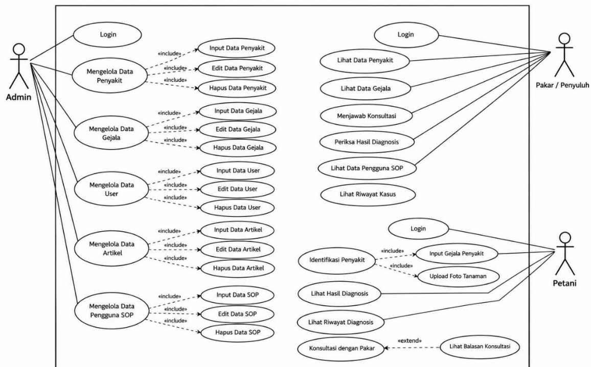
Gambar 3. Use Case Diagram Sistem Manajemen Data Kakao
