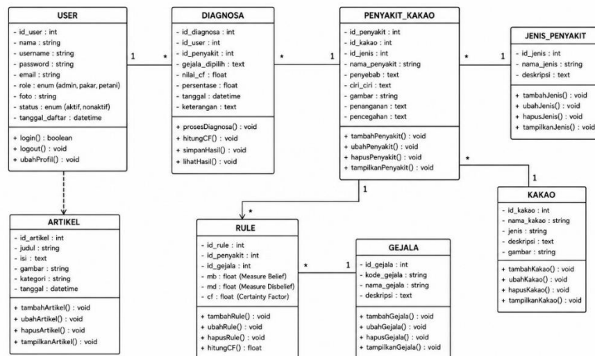
Gambar 5. Class Diagram Sistem Manajemen Data Kakao
